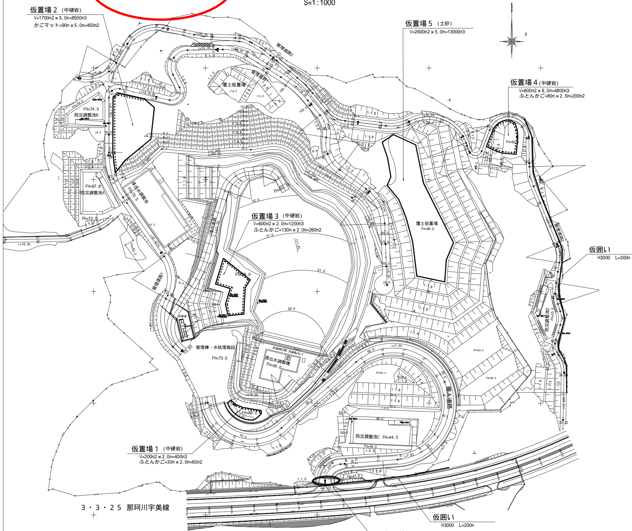
仮置・工用ゲート 平面図 S=1:1000
